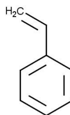
styrene
