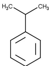
cumene
