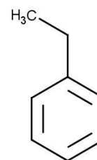
ethylbenzene
