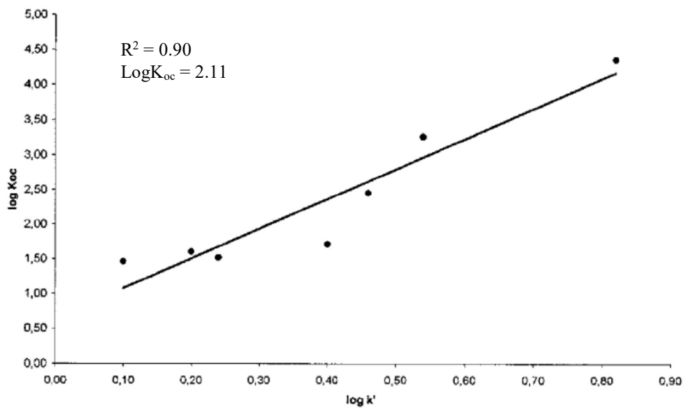
Figure A7.1.3/1-1: \log K_{oc} v \log k'
