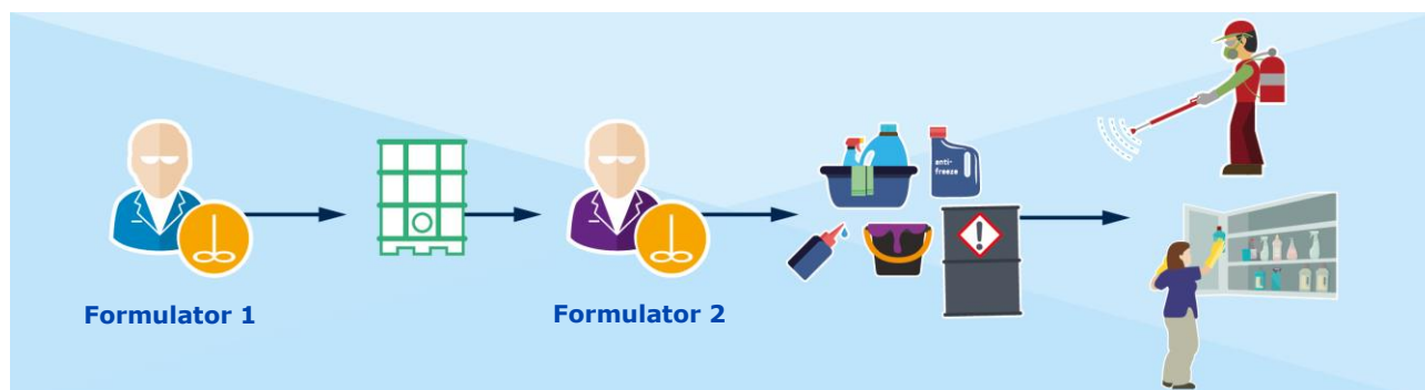
Slika 2. Smjese za daljnje formuliranje koje se upotrebljavaju za formuliranje proizvoda za krajnju uporabu za potrošače, profesionalne krajnje korisnike i/ili krajnje korisnike u industriji
